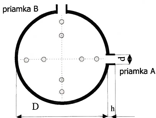
Obrázok č. 3 Prierez potrubia v mieste merania TK8
