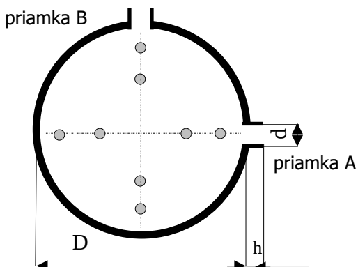
Obrázok č. 5 Prierez potrubia v mieste merania TKG1 a TKG2
